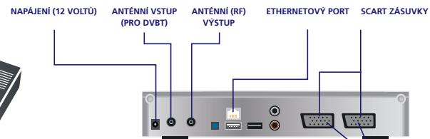
Set-top-box (zezadu)
